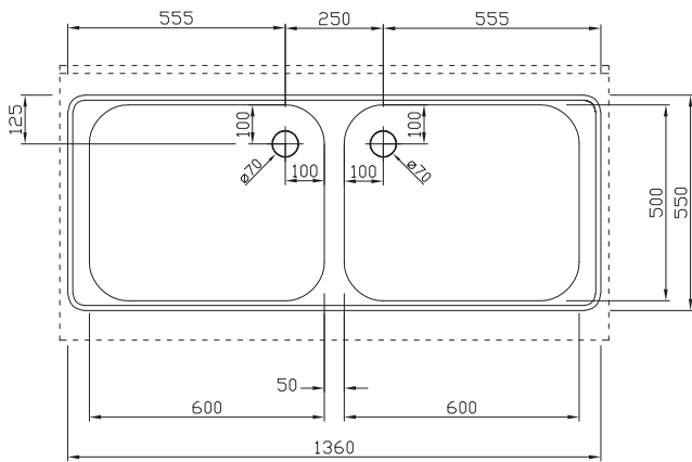
Boven aanzicht
